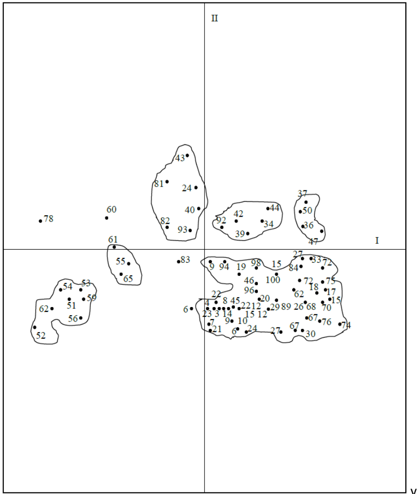
Fig. 2: Species Ordination
