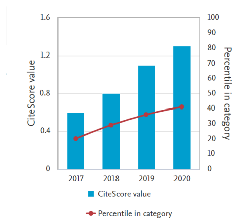
Trend citačního skóre časopisu v rámci kategorie Environmental science – Nature and landscape conservation, kde nám patří 103 příčka ze 177 časopisů (41. percentil)
